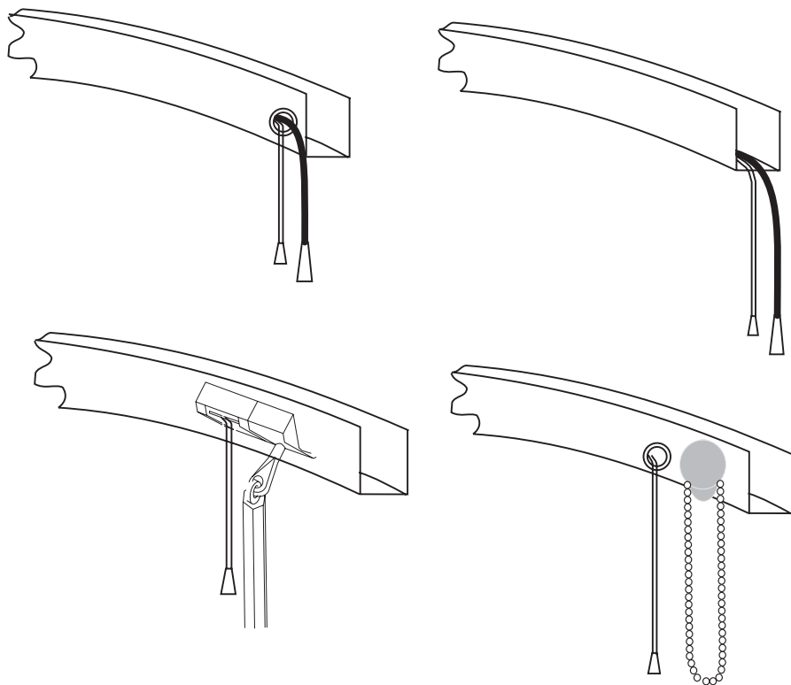
Provedení ovládání obloukových žaluzií
