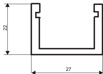
Rozměry horního profilu obloukových žaluzií
